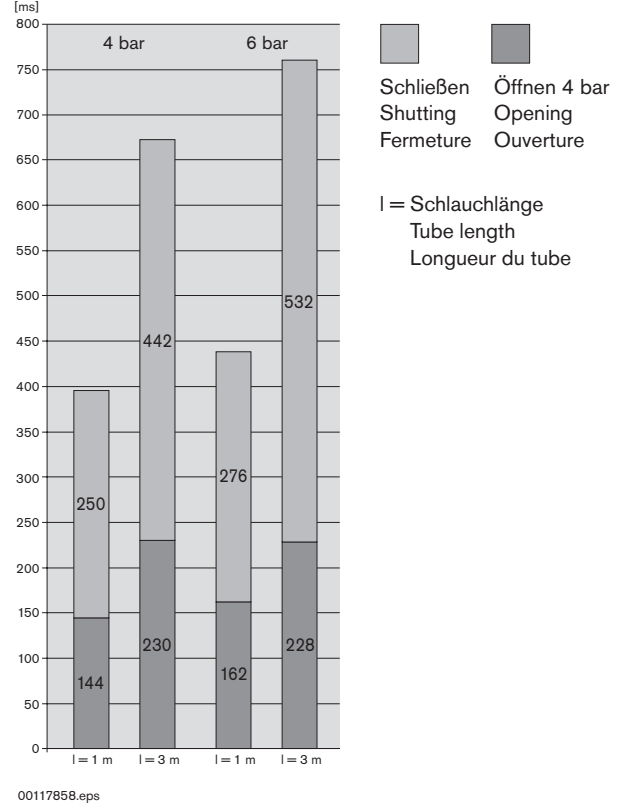
VE 2/L Öffnungs- und Schließzeiten Opening and shutting times Temps d'ouverture et de fermeture
