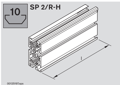
Streckenprofil SP 2/R-H SP 2/R-H conveyor section profile Profilé de section SP 2/R-H
