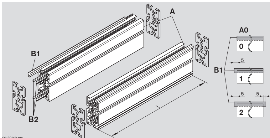
Strecke ST 2/R-V ST 2/R-V section Section ST 2/R-V
