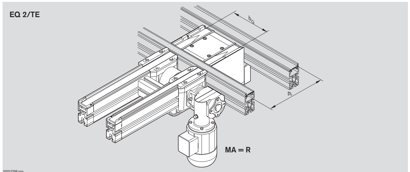
Elektrischer Quertransport EQ 2/TE EQ 2/TE electrical transverse conveyor Convoyeur transversal électrique EQ 2/TE
