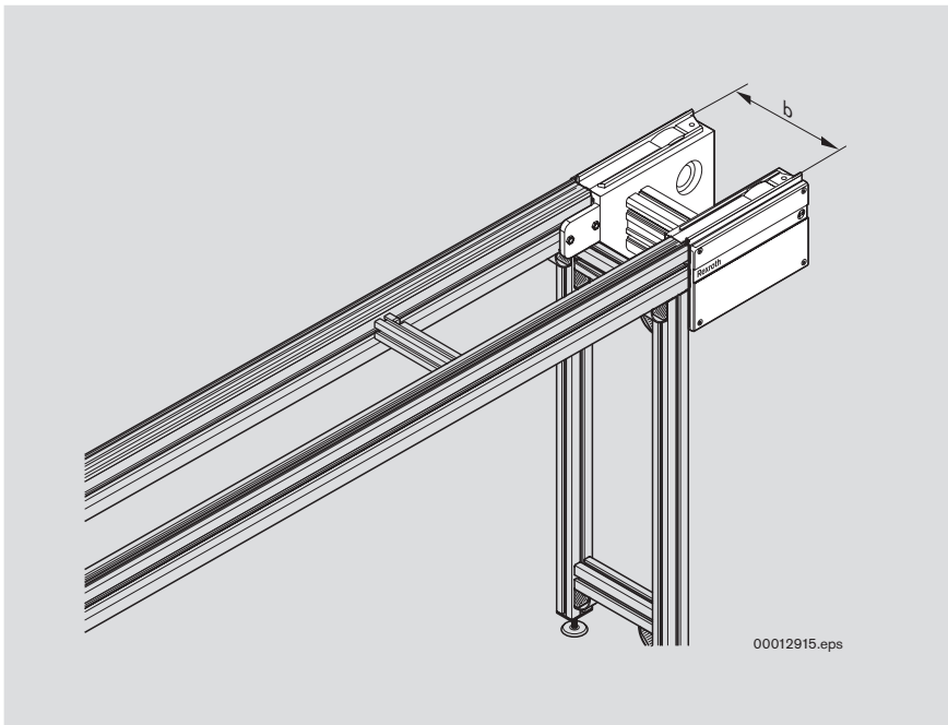
Umlenkung UM 2/B UM 2/B return unit Renvoi UM 2/B
