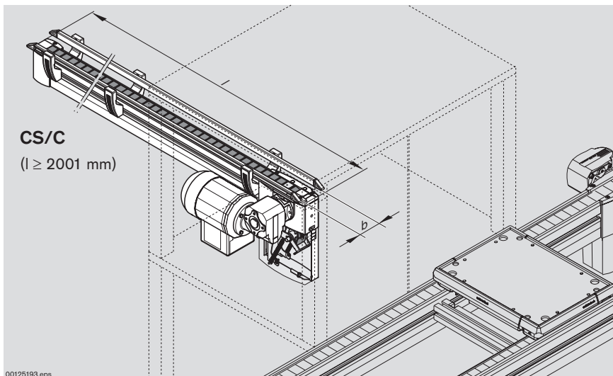
Strecke CS/C Einspur Single-track CS/C section Section CS/C à simple voie
