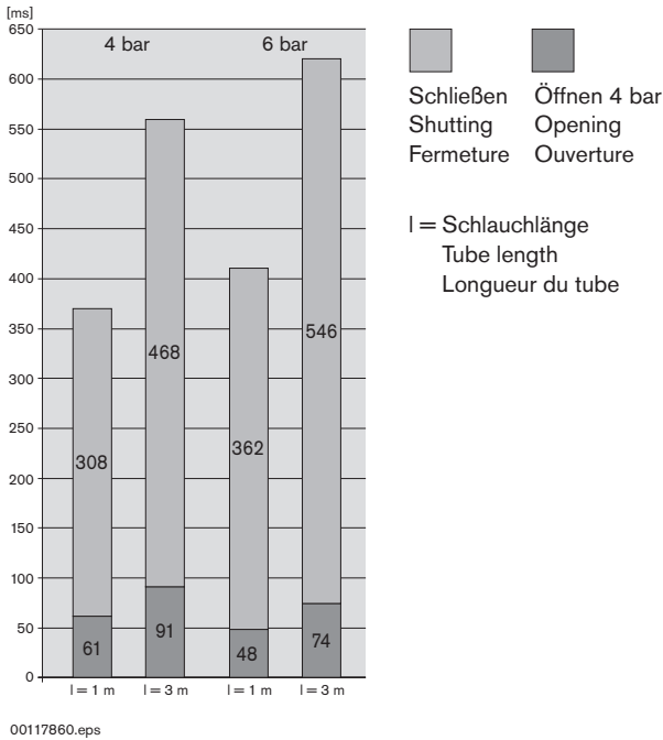
VE 2 Öffnungs- und Schließzeiten Opening and shutting times Temps d'ouverture et de fermeture
