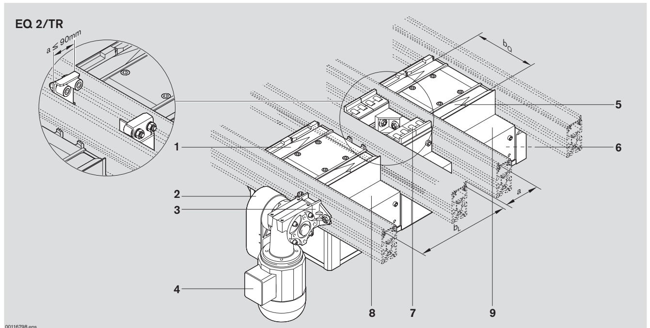
Elektrischer Quertransport EQ 2/TR EQ 2/TR electrical transverse conveyor Convoyeur transversal électrique EQ 2/TR
